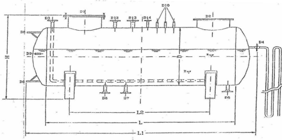
Τεχνικά Στοιχεία Δεξαμενής Τροφοδοσίας Νερού (με στόμιο προσαγωγής απαερωτού & ανθρωποθυρίδα), ΘΕΡΜΟΣΩΛ ΑΤΜΟΛΕΒΗΤΕΣ Α.Ε.
